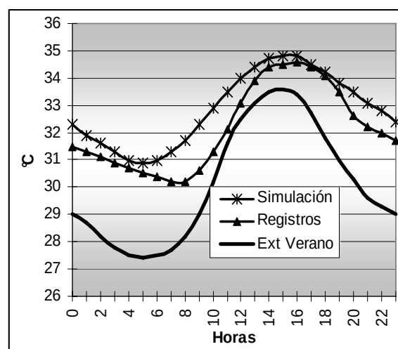
Figura 4. Comparación entre temperaturas exteriores, interiores registradas con HOBO y temperaturas interiores obtenidas con un programa de simulación numérica.
