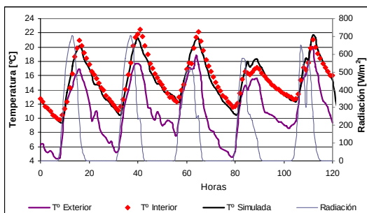
Figura N°10: Resultados del análisis obtenidos con el programa Simedif – mes de agosto
