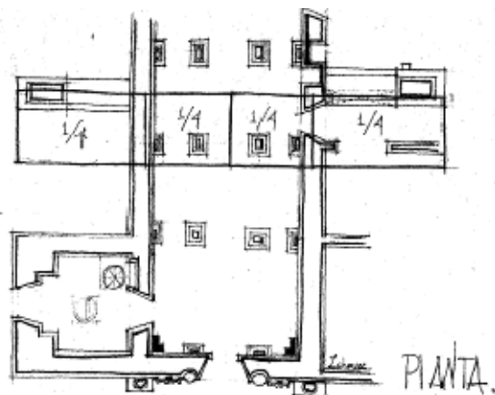
Figura 8. Proporción de los claros del Templo de San Juan Bautista de Tiripetío, Michoacán, México.
