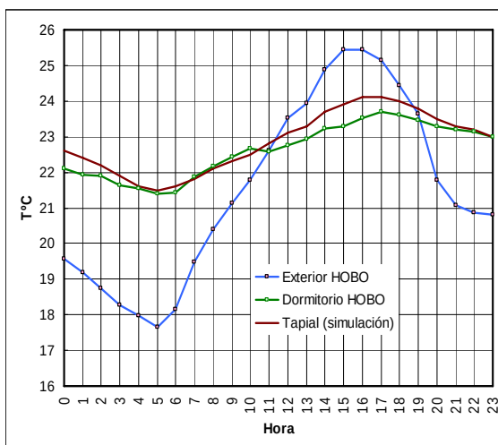
Figura 4. Comparación entre temperaturas exteriores, interiores registradas con HOBO y temperaturas interiores obtenidas con un programa de simulación numérica.
