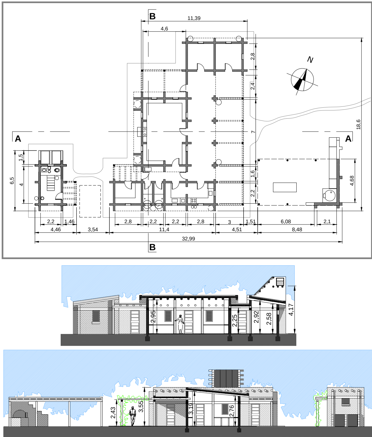
Fig.1. Anteproyecto de la UPRC para Balde de Leyes: planta y cortes.
