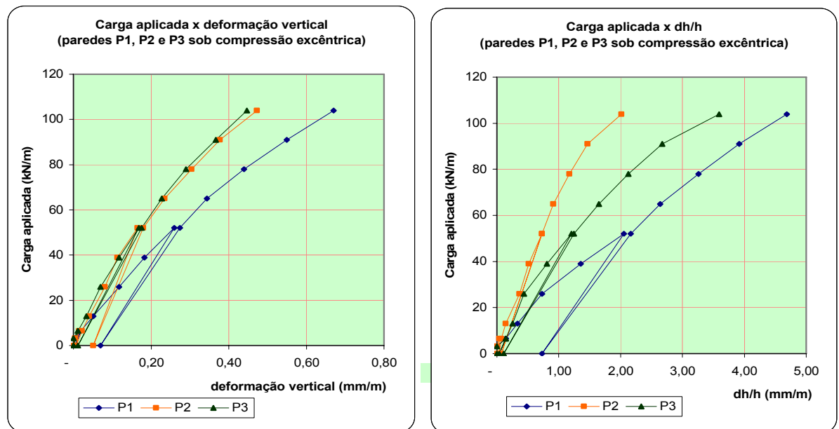
(a) Carga aplicada x deformação vertical
