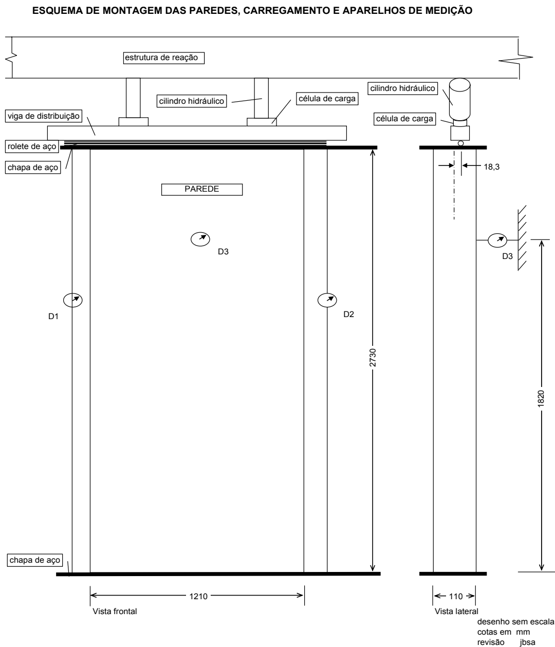
Figura 2 – Esquema de montagem dos instrumentos das paredes
