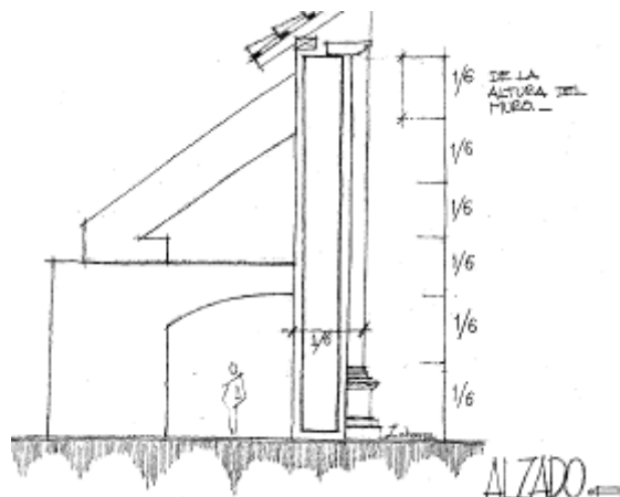
Figura 5. Proporcionamiento según tratado de Vitruvio para obtención del ancho de los muros
