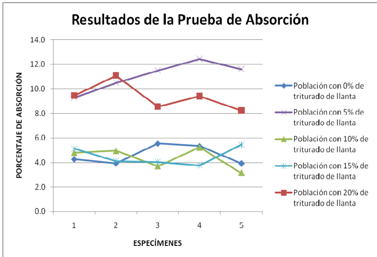
Figura 3 Gráfica del comportamiento de las muestras en la prueba de absorción
