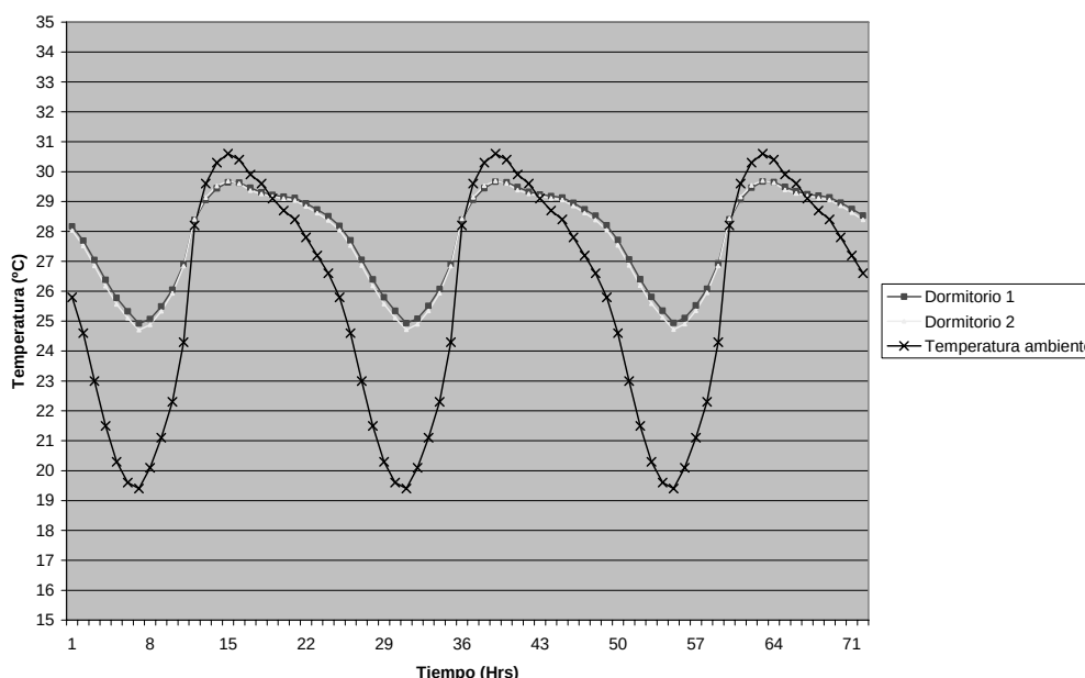
Figura 26: Comportamiento térmico de los locales de la vivienda en relación Temperatura exterior (SIMEDIF [4]).
