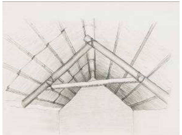
Fig. 3 y 4 Croquis interiores mostrando la disposición de las tijeras y el torillos, vinculadas a las costaneras y la cumbrera.
