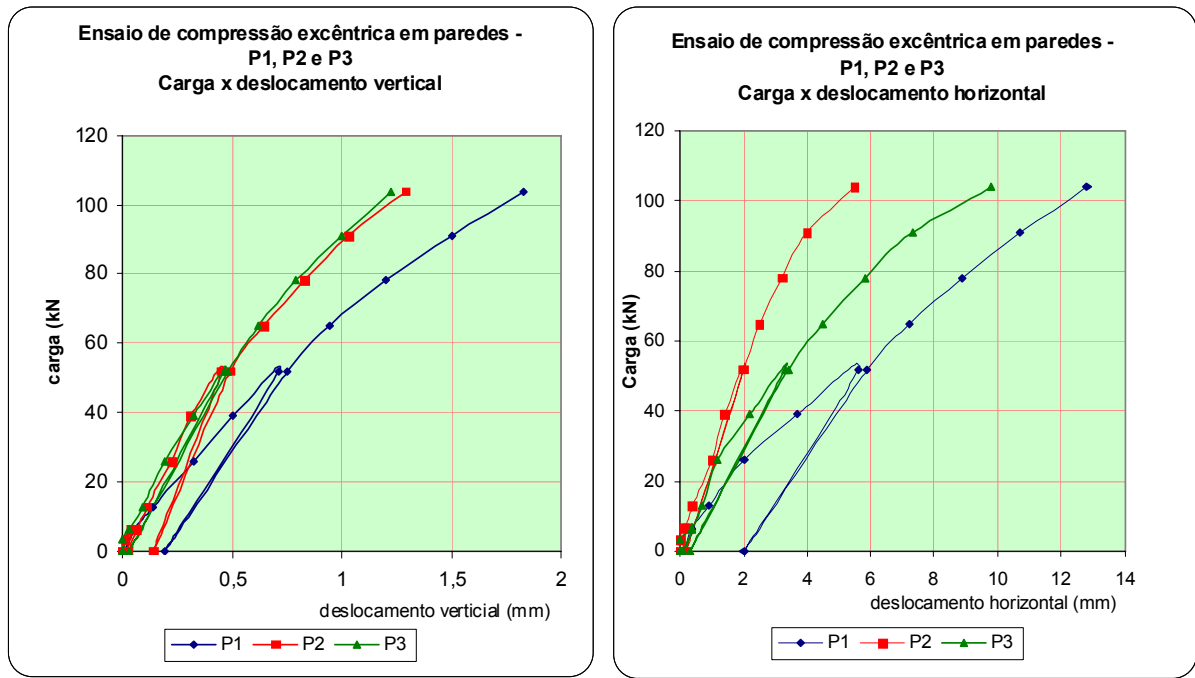
(a) Carga x deslocamento vertical
