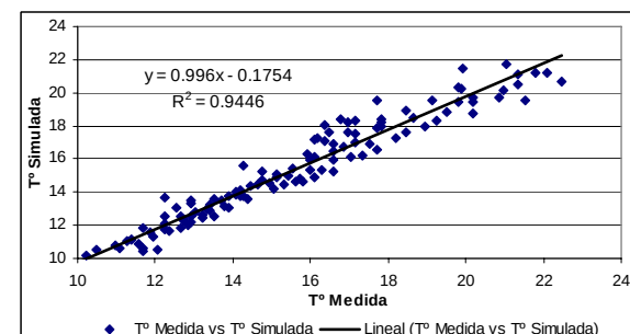
Figura N°11: Correspondencia entre los valores de temperatura medidos vs simulados-agosto
