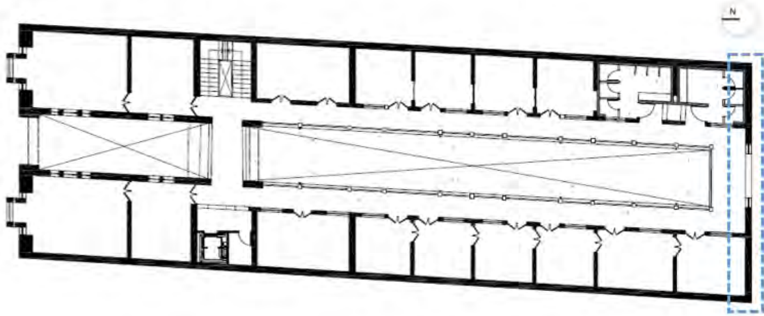
Figura 1. Plano del Pasaje León, planta alta, en donde se señala el muro intervenido. Crédito: Baquero, 2014
