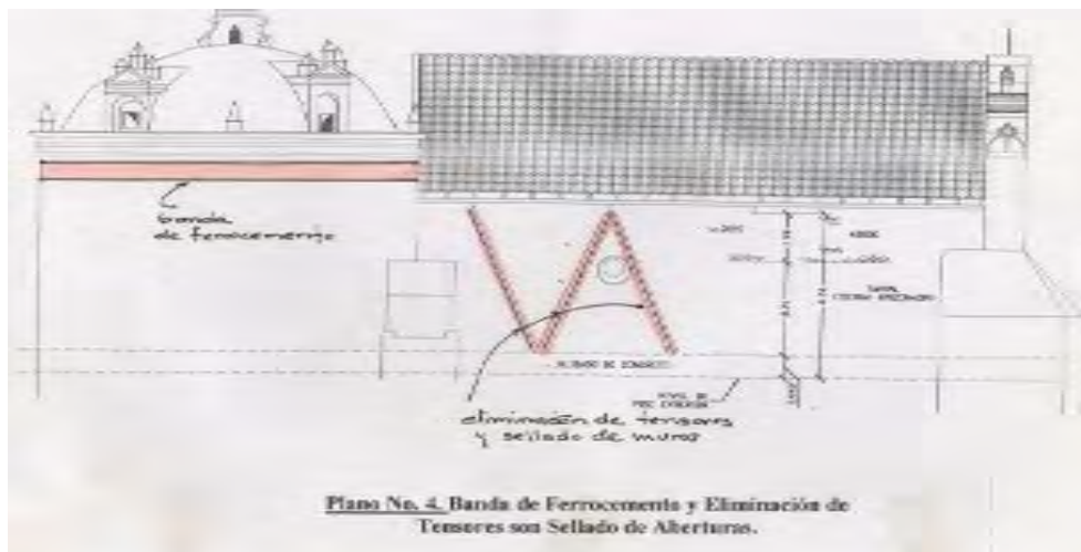
Figura 8. Plano de elevación de fachada lateral sur del templo (Quiñónez, 2002). (observar posición de banda de ferrocemento y ubicación de tensores eliminados)
