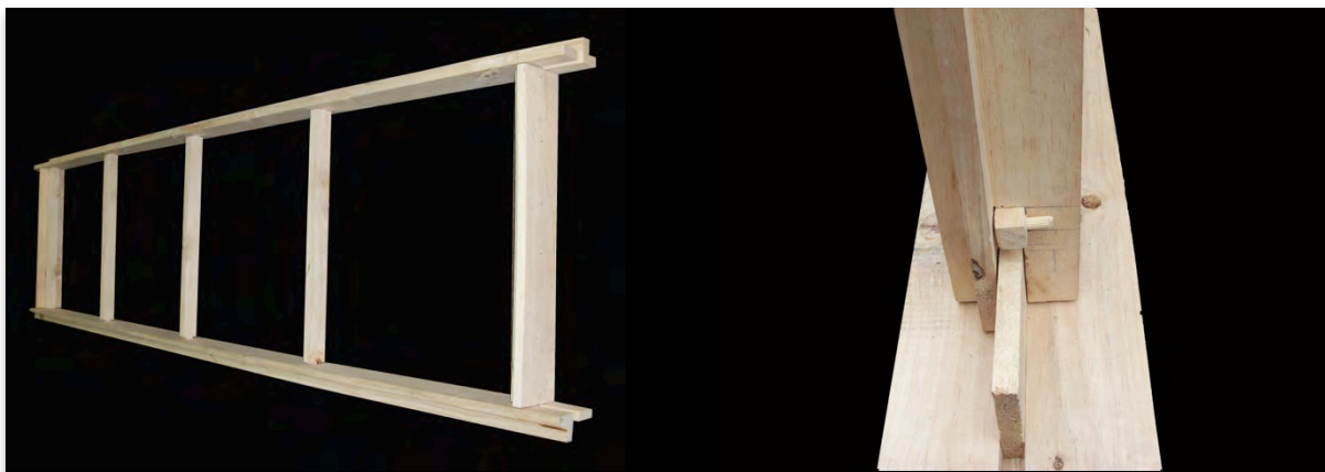
Figura 2 – Imagen de la estructura y detalle de unión con pasadores
