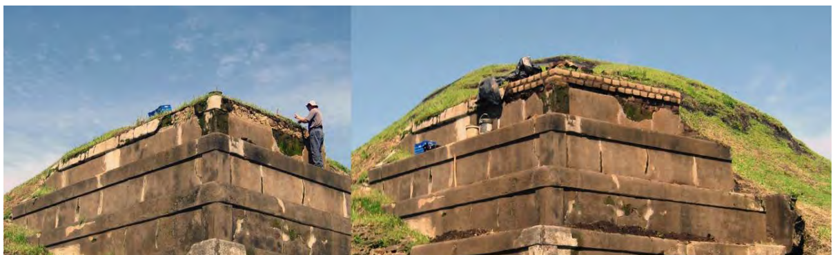
Figura 2 – Esquina Noreste dañada y colocación de adobes para formar la cornisa.
