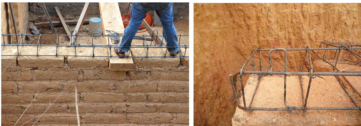
Figura 7. Armado con grapas de acero amarradas a cada 60 cm para anclar la estructura de madera a los muros
