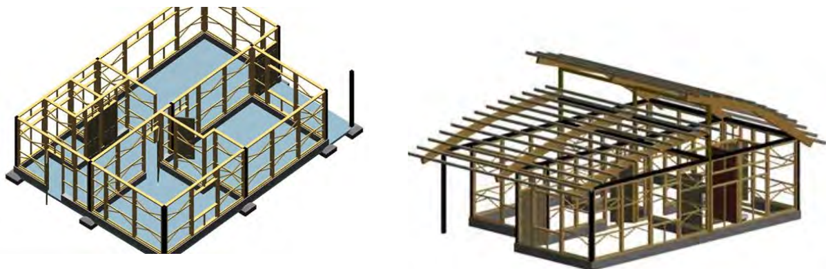
Figura 4- Perspectivas del proyecto arquitectónico semilla (55 m 2 ) - bahareque prefabricado
