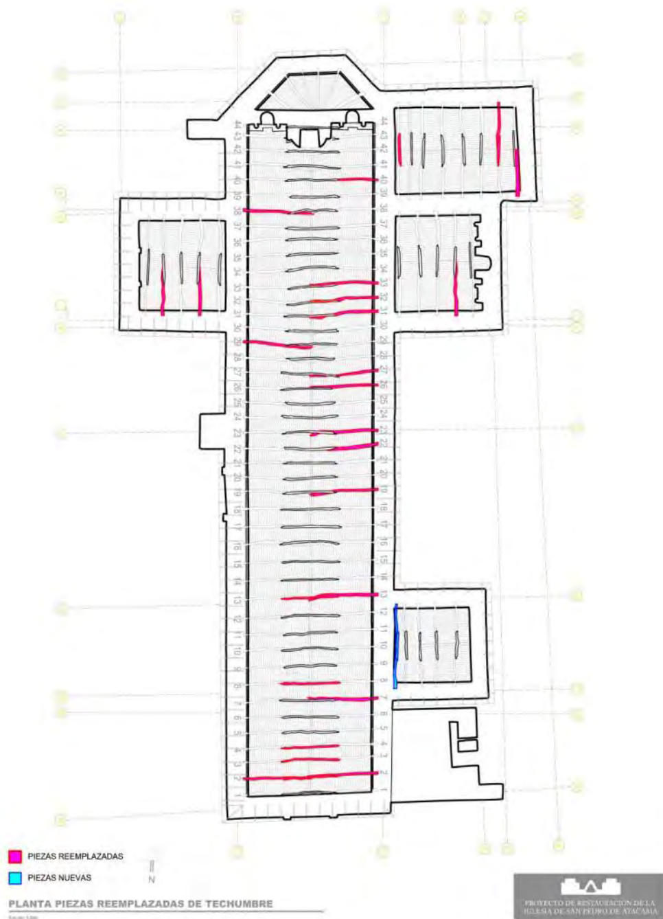
Figura 3. Planta de pares y nudillos reemplazados y piezas nuevas
