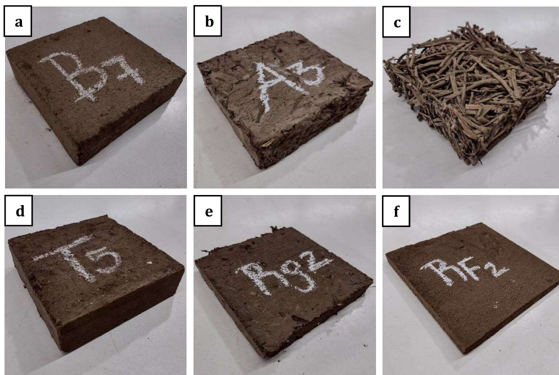
Figura 1: Probetas representativas de las diferentes técnicas constructivas de tierra: a) BTC, b) adobe, c) relleno de quinchá, d) tapia, e) revoque grueso y f) revoque fino
