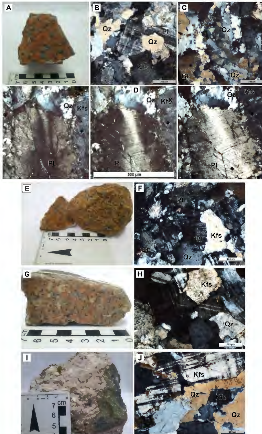
FIGURA 3. Granito Guazunambí: A) Muestra de mano. B, C) Fotomicrografías con luz polarizada. D) Cristal de plagioclasa mostrando extinción ondulante y la macla polisintética deformada. Granito Policlínica: E) Muestra de mano. F) Fotomicrografías con luz polarizada. Granito Yermal - Facies Monzogranito Rosado: G) Muestra de mano. H) Fotomicrografías con luz polarizada. Granito Yermal - Facies Leucogranito Blanco: I) Muestra de mano. J) Fotomicrografías con luz polarizada. Abreviaciones minerales siguiendo a Siivola & Schmid, (2007)
