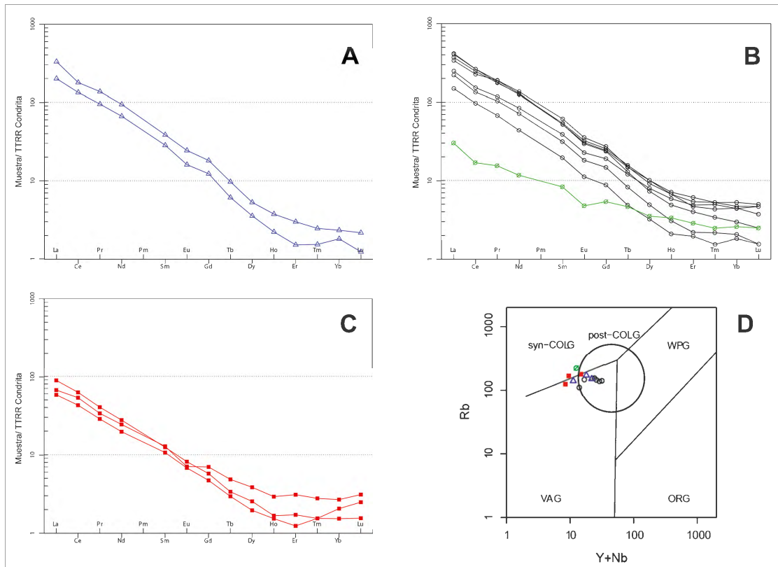
FIGURA 10. Diagrama tipo spider. (A), (B) y (C) normalizado a condrita (Boynton, 1984). (D) Diagrama de discriminación tectónica de Pearce (1995) Rb vs Y+Nb. Granitos Guazuambí \Delta , Policlínica \blacksquare , Yermal O y facies de leucogranito blanco \circ . FIGURE 10. Spider diagram. (A), (B) and (C) normalized to chondrite (Boynton, 1984). (D) tectonic discrimination diagram Rb vs Y + Nb (Pearce 1995). Granites Guazuambí \Delta , Policlínica \blacksquare , Yermal O and white leucogranite facies \circ .
