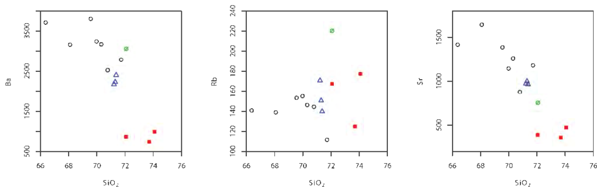
FIGURA 8. Diagramas Harker de elementos traza (ppm) versus SiO 2 (% en peso) para los tres granitos. Granitos Guazunambí \Delta , Policlínica \blacksquare , Yermal \circ y facies de leucogranito blanco \circ .
