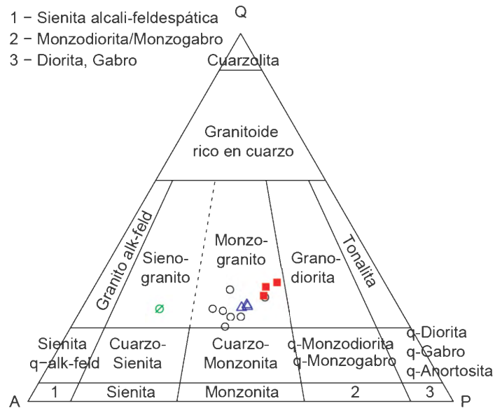
FIGURA 4. Diagrama QAP de (Streckeisen, 1976). Granitos Guazunambí \Delta , Policlínica \blacksquare , Yermal O y facies de leucogranito blanco \circ .
