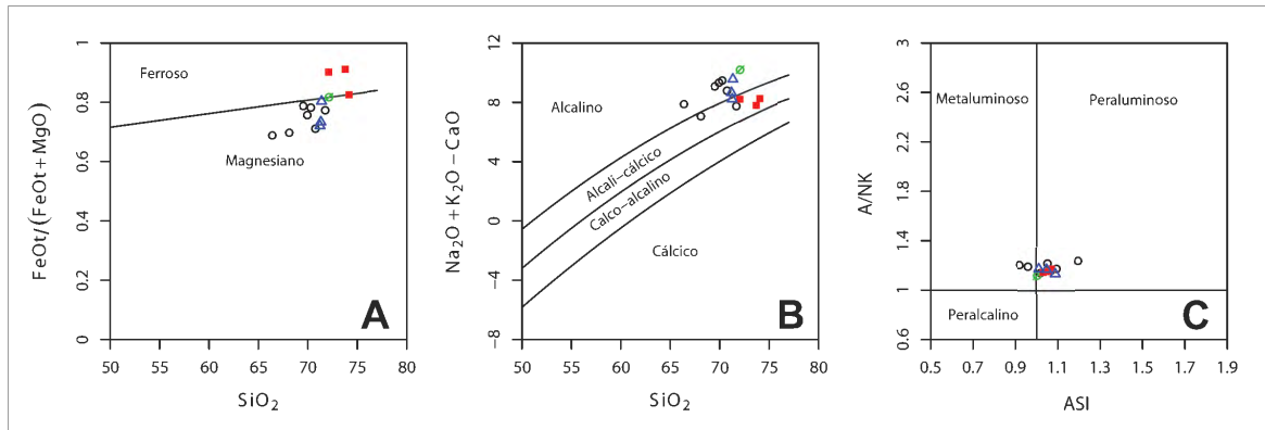
FIGURA 6. (A) Diagrama \text{FeOt} / (\text{FeOt} + \text{MgO}) vs \text{SiO}_2 de Frost et al. (2001). (B) Diagrama \text{Na}_2\text{O} + \text{K}_2\text{O} - \text{CaO} vs \text{SiO}_2 de Frost et al. (2001) (C) Diagrama de Shand (1943), modificado por Frost et al. (2001). Granitos Guazunambí \Delta , Policlínica \blacksquare , Yermal \circ y facies de leucogranito blanco \circ .
