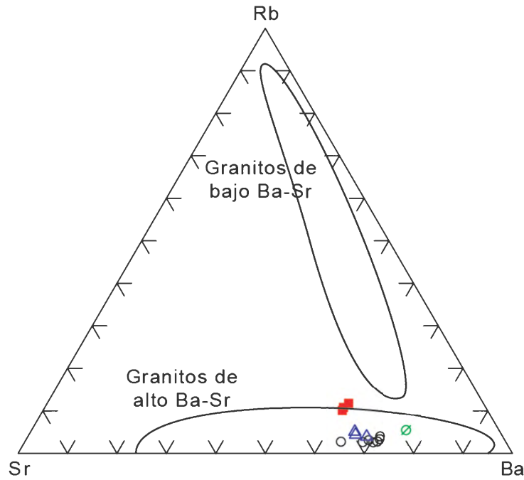
FIGURA 9. Diagrama de Tarney y Jones (1994). Granitos Guazuambí \Delta , Policlínica \blacksquare , Yermal O y facies de leucogranito blanco \circ . FIGURE 9. Rb-Ba-Sr diagram (Tarney and Jones 1994). Granites Guazuambí \Delta , Policlínica \blacksquare , Yermal O and white leucogranite facies \circ
